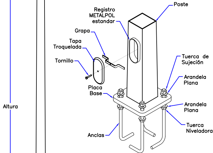
Detalle 1
