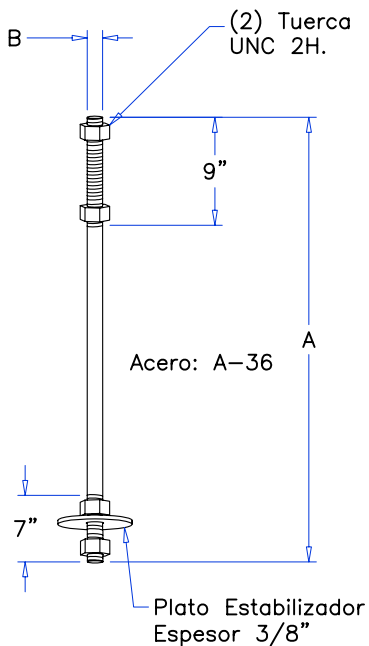
Detalle de Ancla
