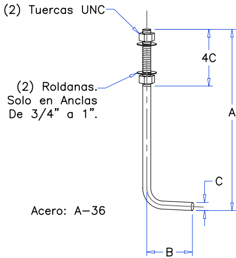
Detalle de Ancla
