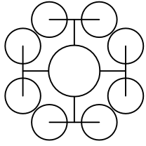
Canastilla Radial Para 8 Luminarias 8 - m p c a n r - 2
